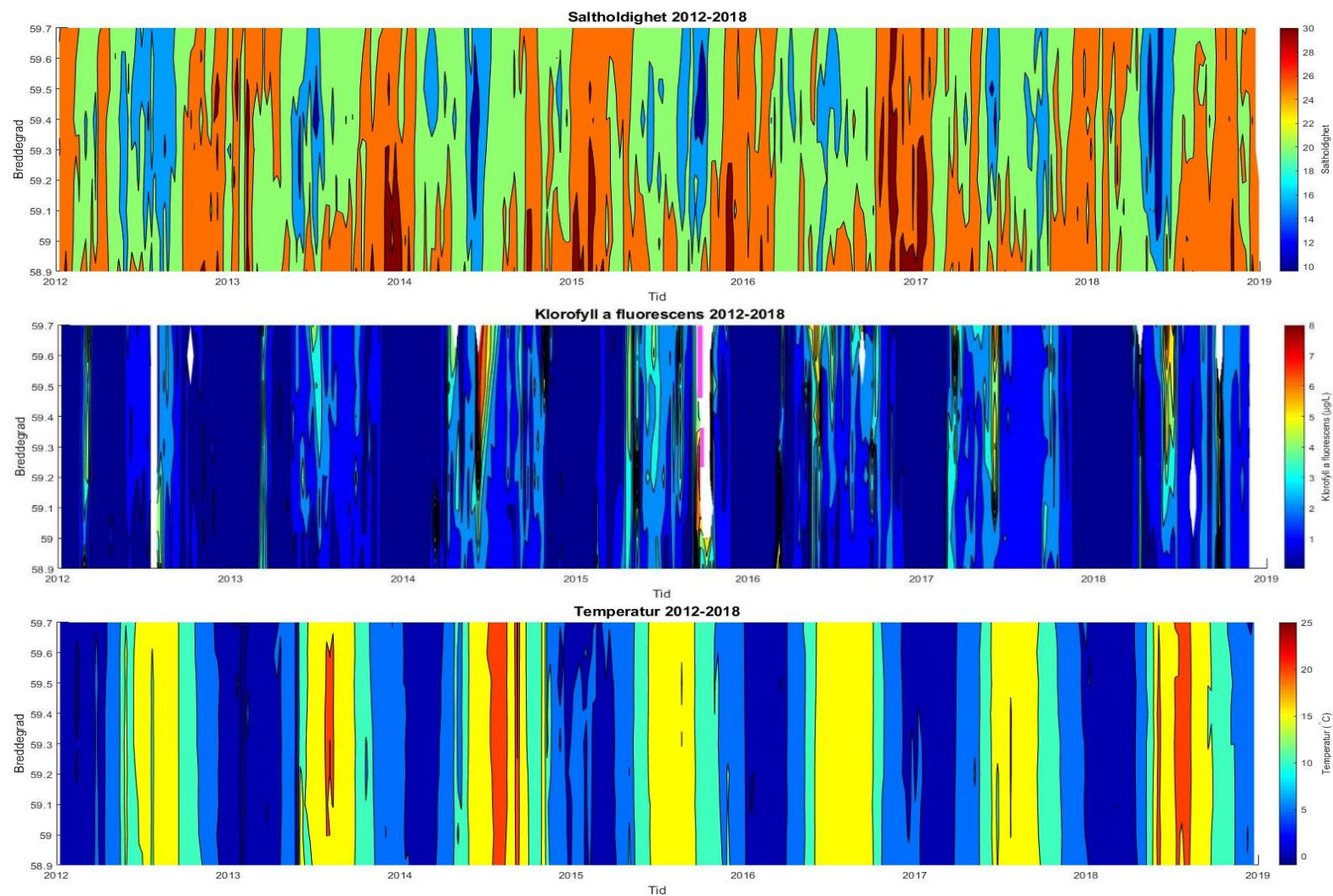
Figur 12. Temperatur, klorofyll a fluorescens og saltholdighet langs ferrybox-ruten (y-akse) i 2012-2018. For klorofyll-a fluorescens ble det kun plottet verdier under 10 \mu\text{g/L} , mens rosa markering viser når det har vært høyere biomasse; kun en kort periode høsten 2015, opp mot 14 \mu\text{g/L} .
