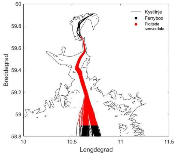
Figur 11. Transekt for MS Color Fantasy med Ferrybox. Figuren viser loggede ruter i perioden 2012-2018. Den røde delen av rutene er området som det er vist data for.
