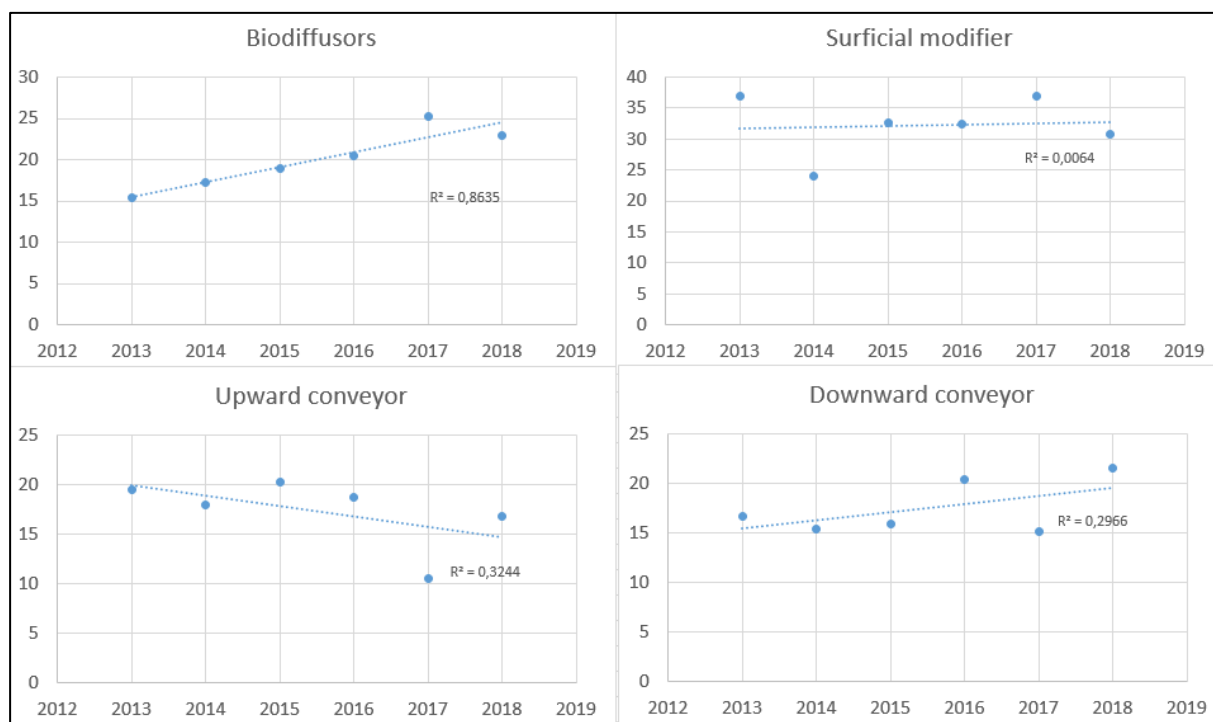
Figur 30 Endring av prosentandelen for kategorier innen egenskapen sediment reworking på stasjon A05 (BT40) i perioden 2013-2018.
