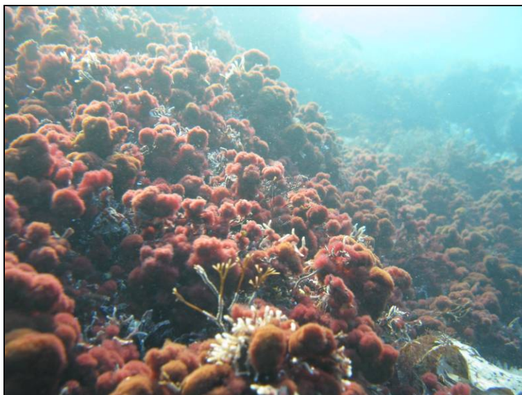
Figur 12. Undervannsfoto fra stasjon G26 Rauerkalven i 2010. Området på bildet er dominert av rødalgen Rødlo ( Trailiella intricata ).
