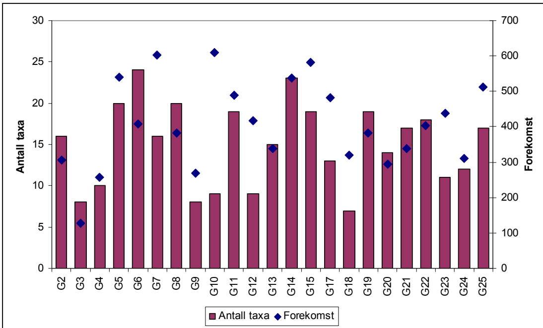
Figur 8. Antall taxa og samlet forekomst (antall ruter hver art ble funnet i) for alger på hver av fjærestasjonene på nedre nivå i 2010 (for stasjonsplassing se Figur 3 ).
