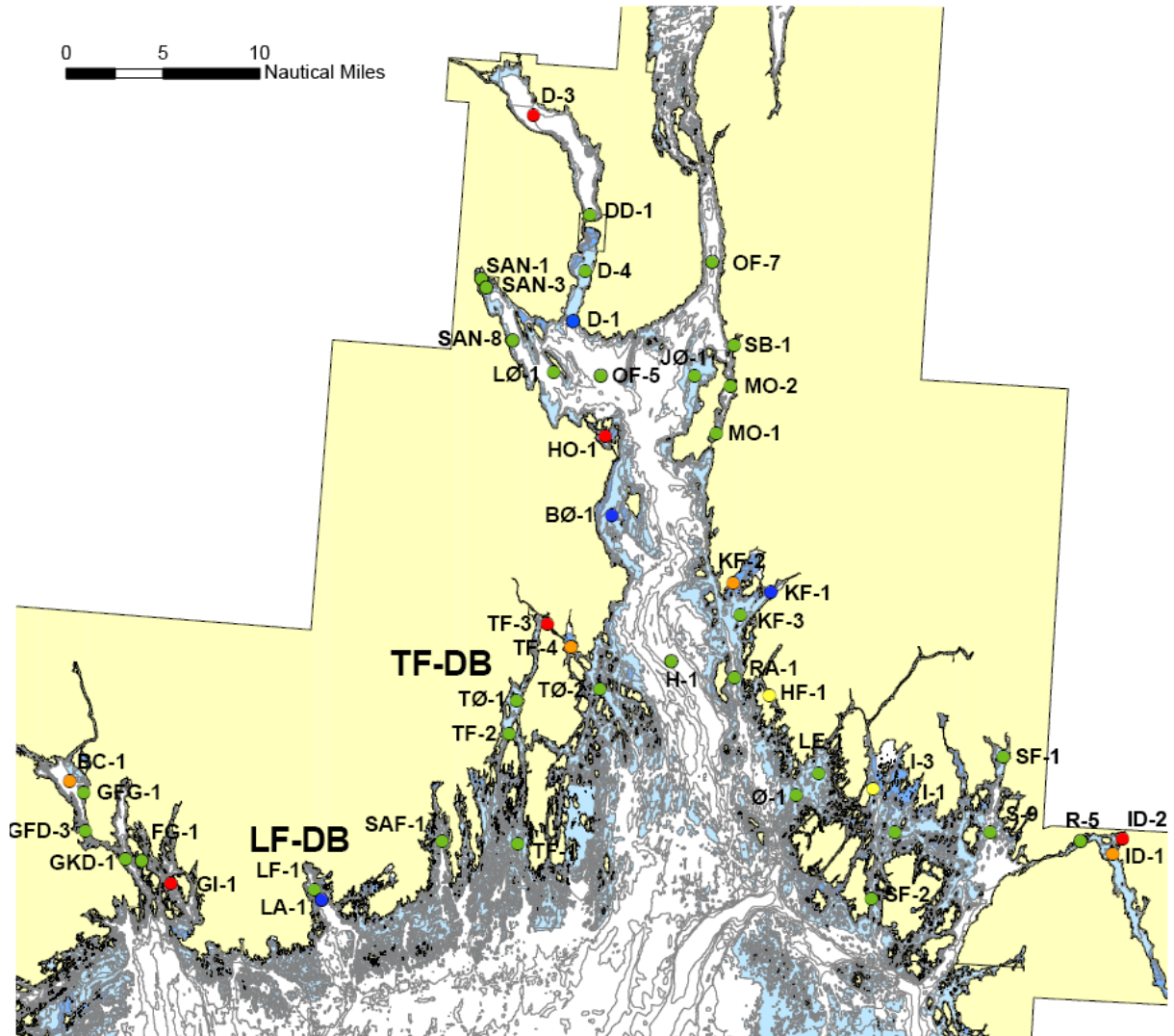
Figur 5. Tilstandsklasser for bløtbunn i henhold til BHQ-indeksen (SPI, Rosenberg m. fl. 2004) fra alle stasjoner i området som ble innsamlet i 2010, se Tabell 2 . Utvidet registrering og analyse av bilder ble utført langs dybdegradient i Larviksfjorden (LF-DB) samt noen stasjoner på ulike dyp ved Tønsberg (TF-DB), se Tabell 1 . Stasjonsnavn i Vedlegg A.
