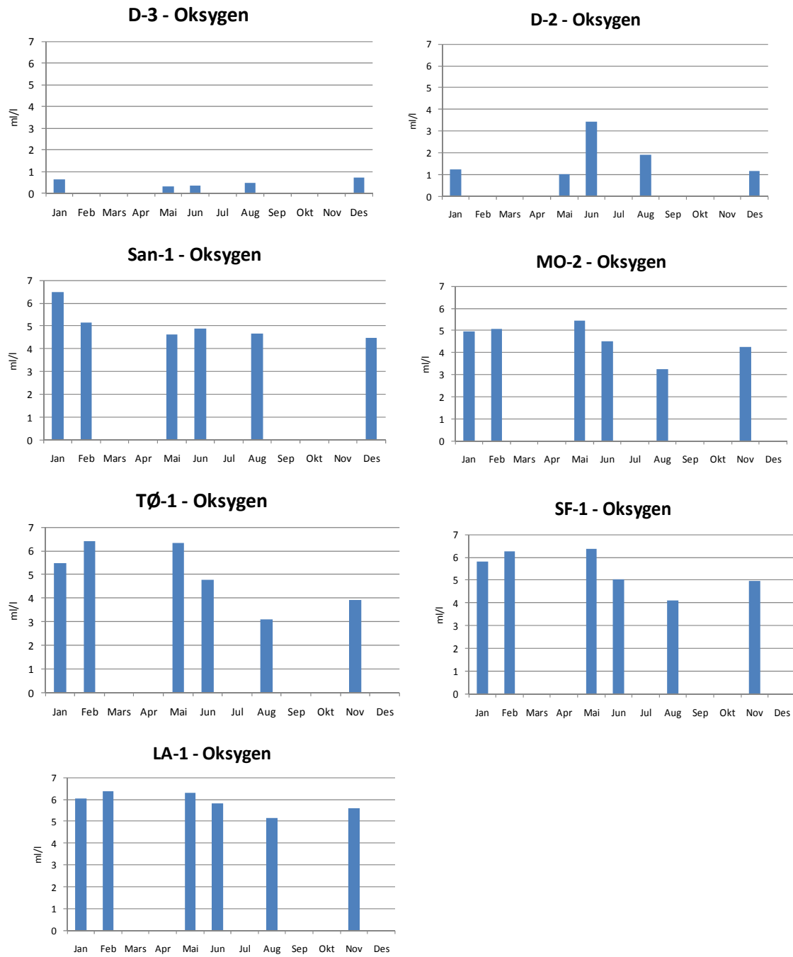
Figur 13. Oksygenmengden i dypeste dyp ved stasjonene i "randsonen" i 2009. For koder se tabell .
