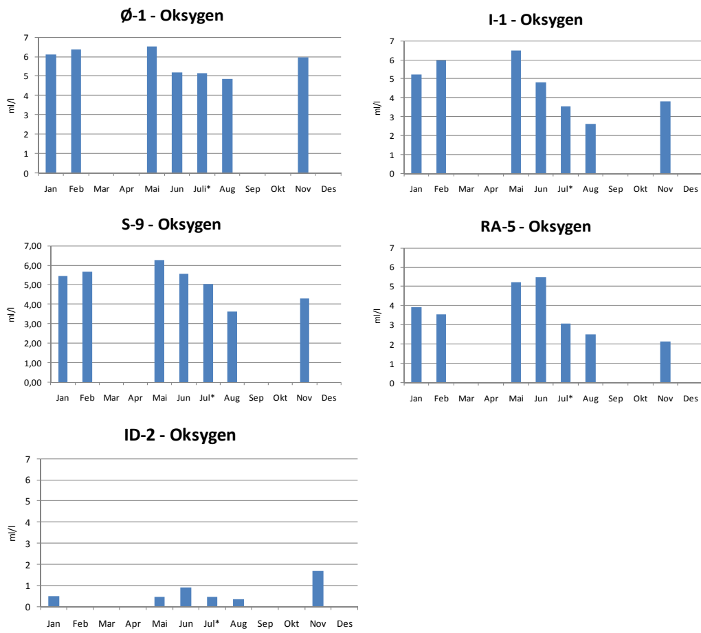
Figur 14. Oksygenmengden i dypeste dyp ved stasjonene i ”randsonen” i 2009. For koder se tabell 1.
