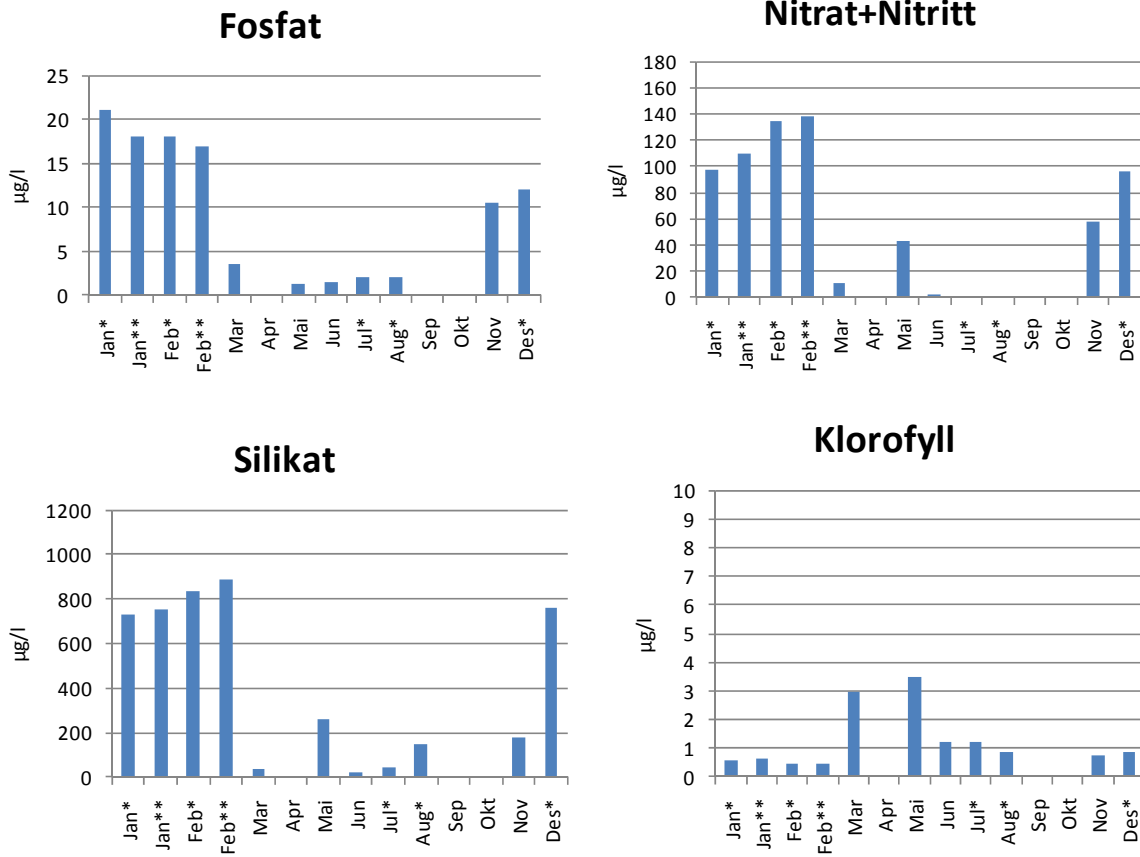
Figur 21. Data fra 5 meter dyp for parameterne Fosfat, Nitrat+Nitritt, Silikat og Klorofyll a ved stasjon "OF-2" 2009.
