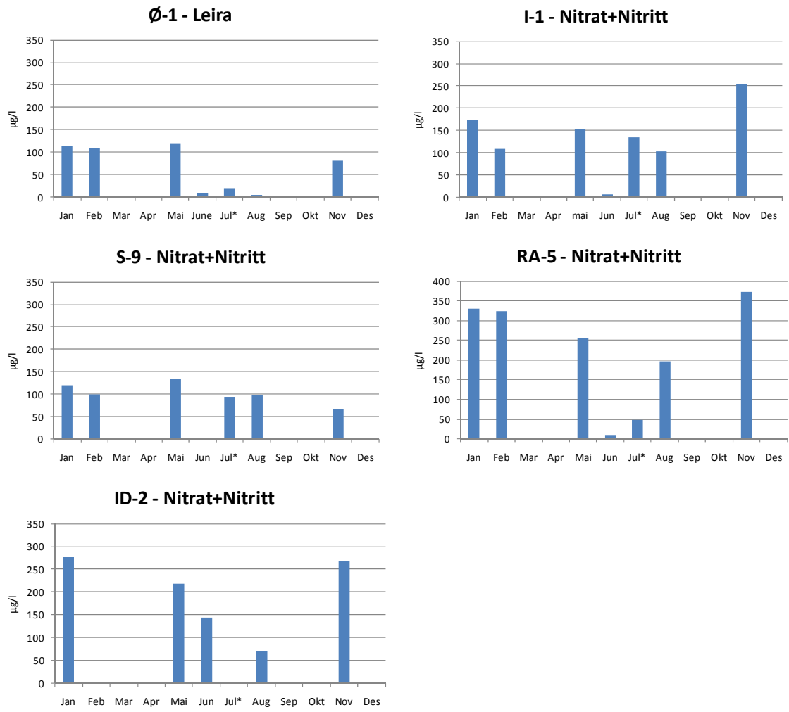
Figur 12. Nitrat + Nitritt konsentrasjonen ved "randstasjonene" 2009. For koder se tabell 1.
