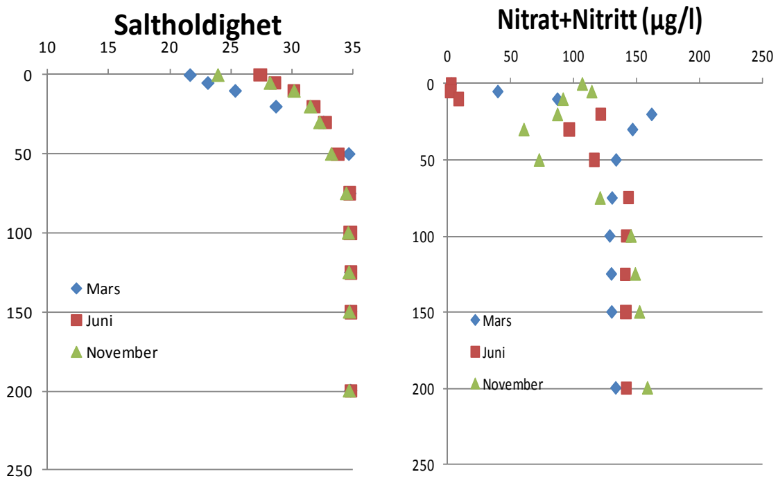
Figur 19. Vertikalprofiler av saltholdighet og Nitrat + Nitritt konsentrasjonen ved stasjonen "OF-7" i mars, juni og november 2009.
