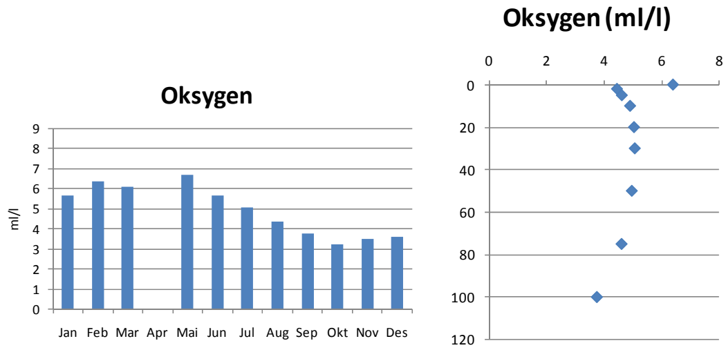
Figur 10. Utviklingen av oksygen i bunnvannet ved "Langesundfjorden" og en vertikal profil av oksygenmengden i september 2009. Data hentet fra Data hentet fra SFT prosjektet "Miljøovervåking av sukkertare" og fra Havforskningsinstituttets overvåkningsprogram i Grenland.
