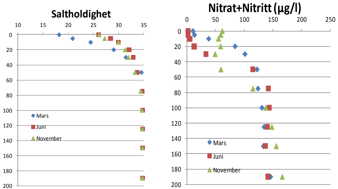
Figur 17. Vertikalprofiler av saltholdighet og Nitrat + Nitritt konsentrasjonen ved stasjonen "OF-4" i mars, juni og november 2009.
