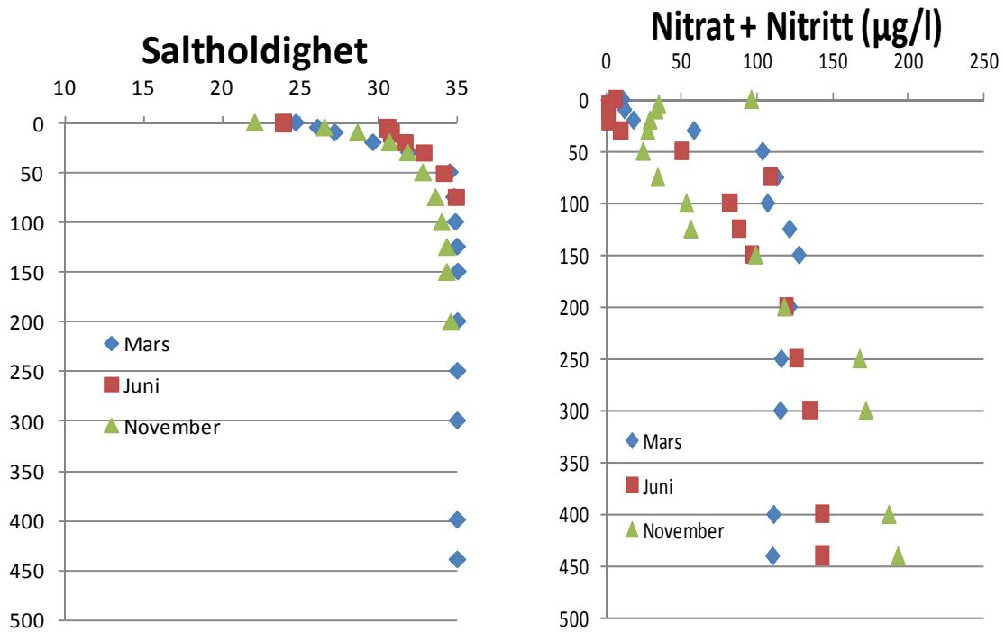
Figur 15. Vertikalprofiler av saltholdighet og Nitrat + Nitritt konsentrasjonen ved stasjonen "OF-1" i mars, juni og november 2009.
