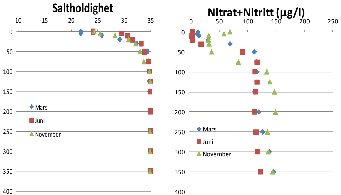
Figur 16. Vertikalprofiler av saltholdighet og Nitrat + Nitritt konsentrasjonen ved stasjonen "OF-2" i mars, juni og november 2009.
