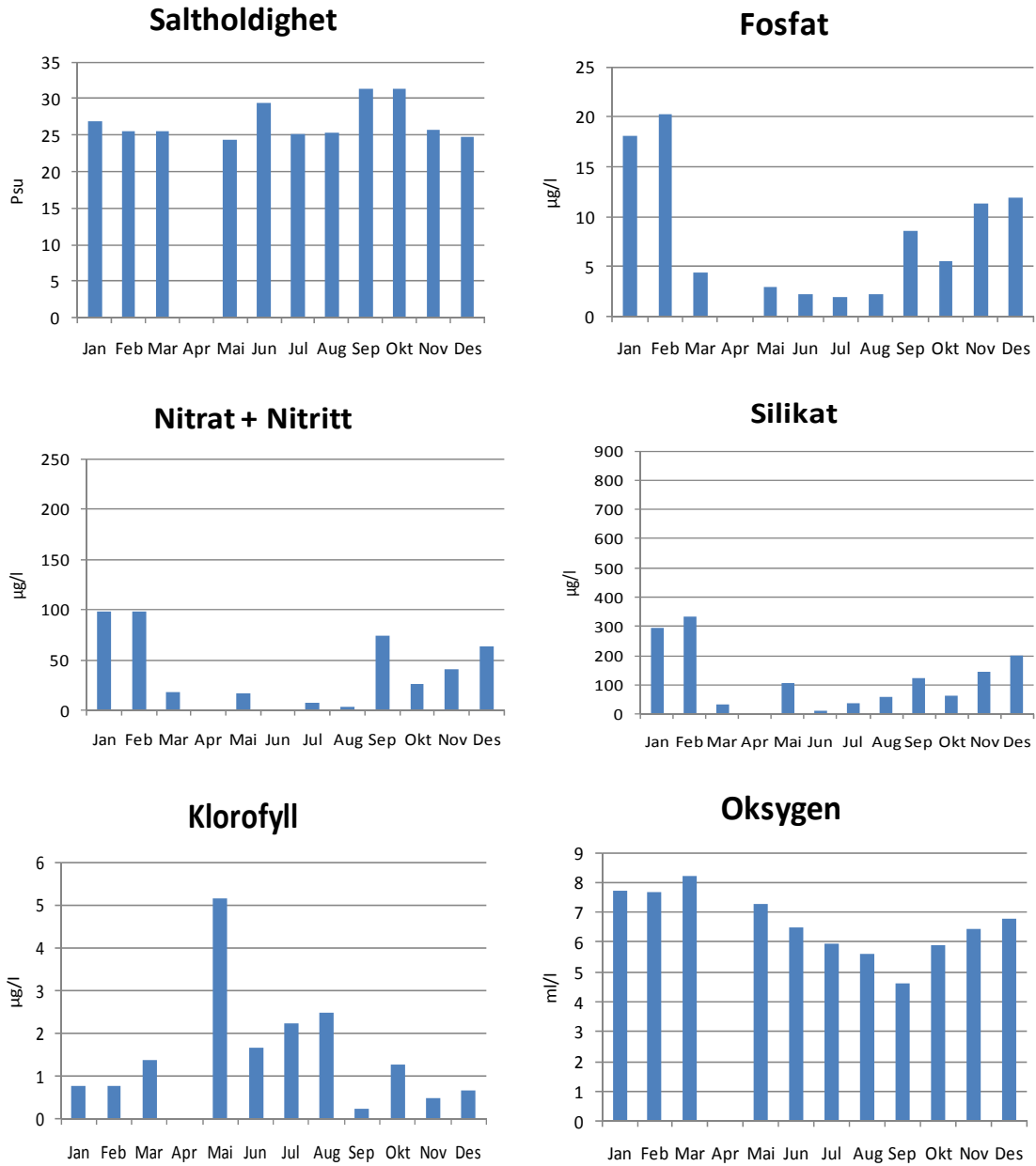
Figur 9. Saltholdighet, Fosfat, Nitrat + Nitritt, silikat, klorofyll a og oksygen i 5 meters dyp ved stasjonen "Langesundfjorden" i 2009. Data hentet fra Data hentet fra SFT prosjektet "Miljøovervåkning av sukkertare" og fra Havforskningsinstituttets overvåkningsprogram i Grenland.
