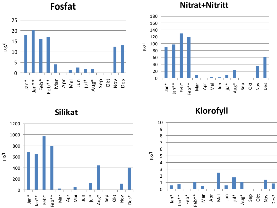
Figur 20. Data fra 5 meter dyp for parameterne Fosfat, Nitrat+Nitritt, Silikat og Klorofyll a ved stasjon "OF-1" 2009.
