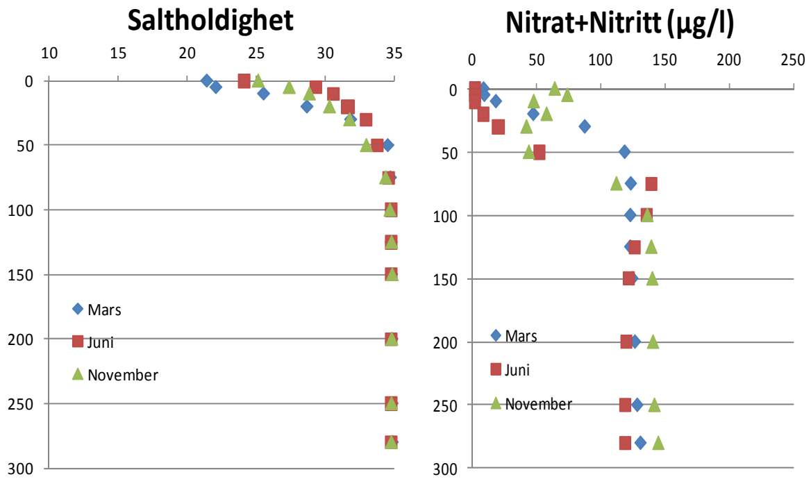
Figur 17. Vertikalprofiler av saltholdighet og Nitrat + Nitritt konsentrasjonen ved stasjonen "OF-4" i mars, juni og november 2009.
