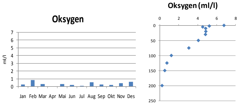
Figur 8. Utviklingen av oksygen i bunnvannet ved "Håøyfjorden" og en vertikal profil av oksygenmengden i september 2009. Data hentet fra SFT prosjektet "Miljøovervåking av sukkertare" og fra Havforskningsinstituttets overvåkningsprogram i Grenland.
